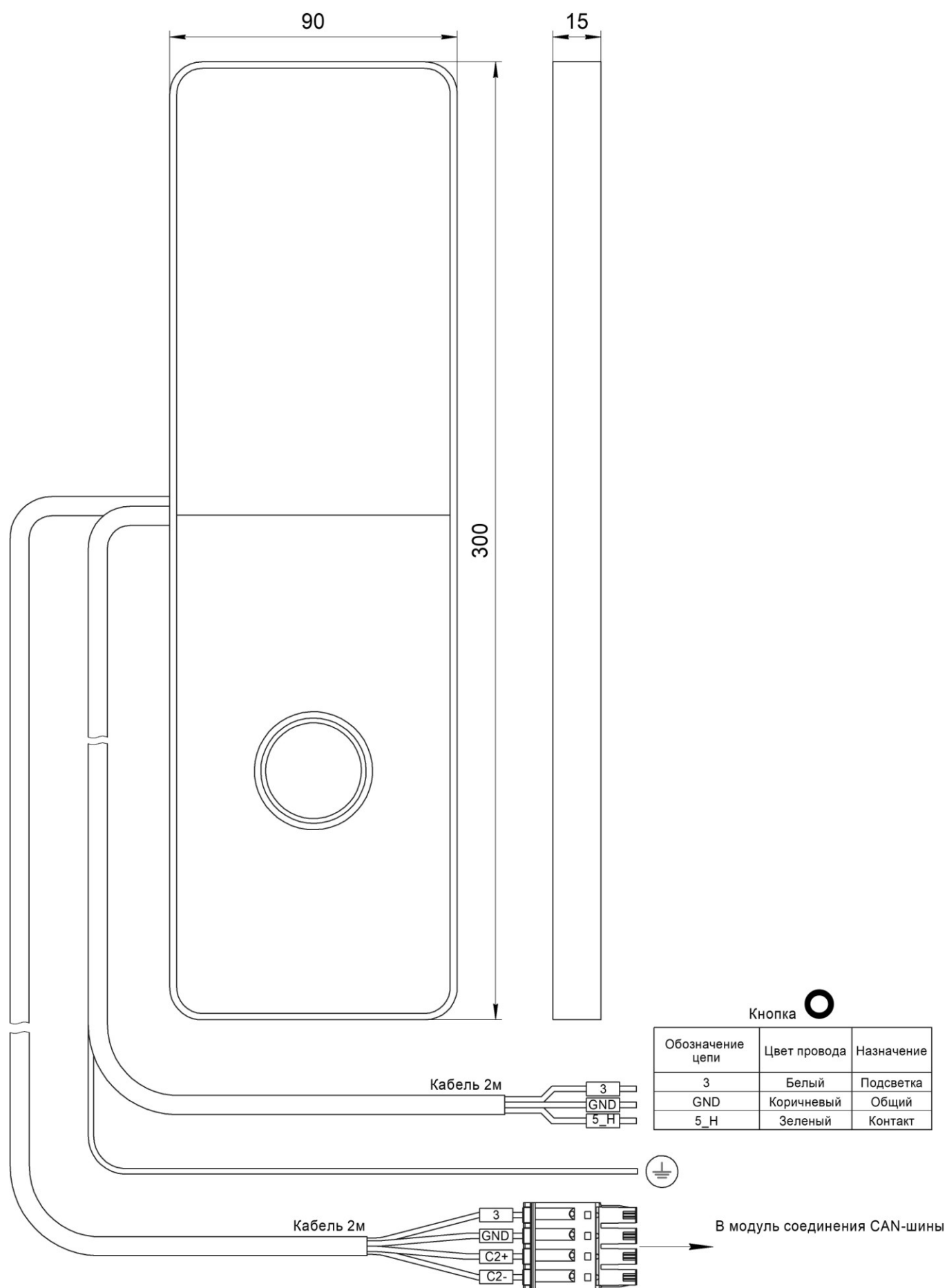
Рис.1 Внешний вид Вызывной пост ОНИКС НШЕК.468381.014
